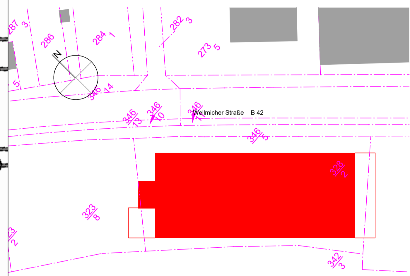
Lageplan M 1:500
